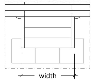
Stairs Detail Scale: 1:50
