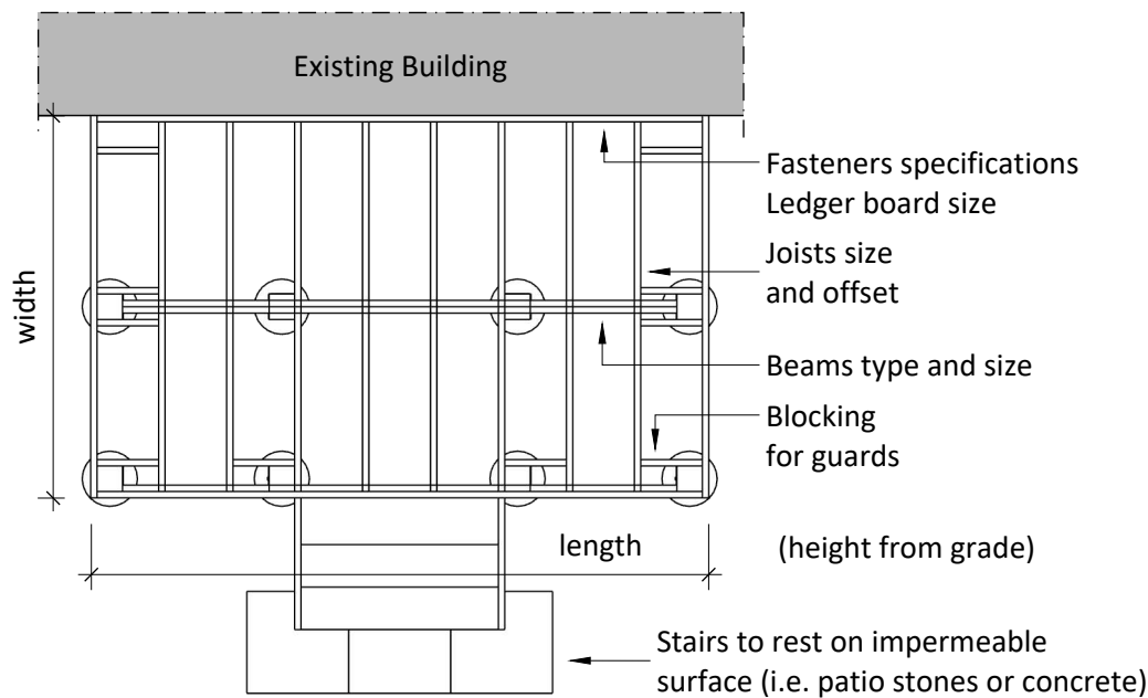
Floor Plan Scale: 1:50
